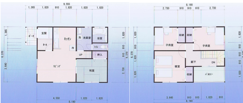
1F 平面図
