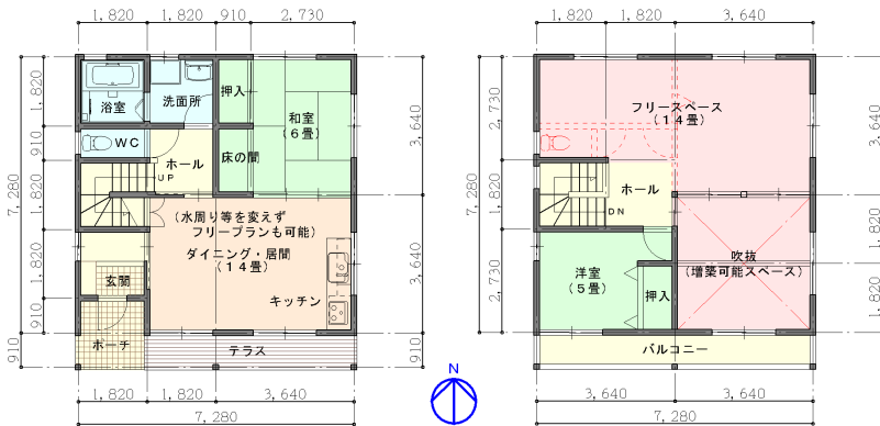
1階平面図
