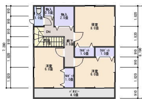
2階平面図
