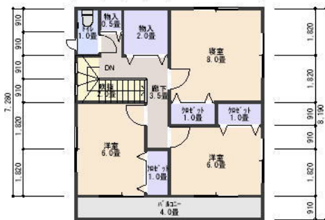
2階平面図
