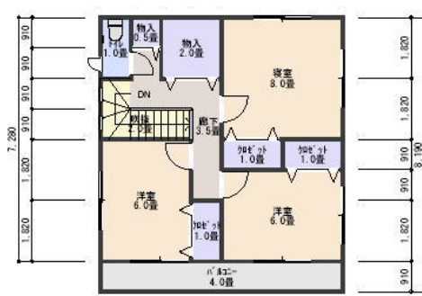
2階平面図
