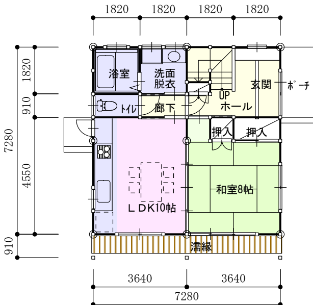
1階平面図 S=1/150
