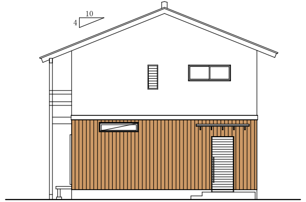
東立面図 S=1/150
