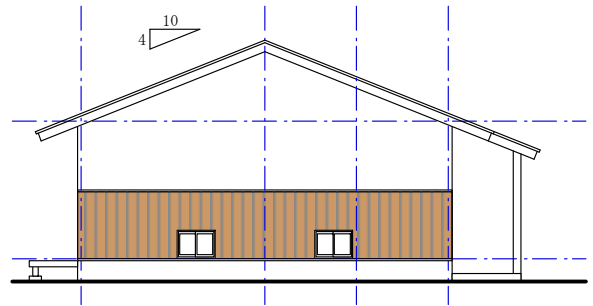
東立面図 S=1/150
