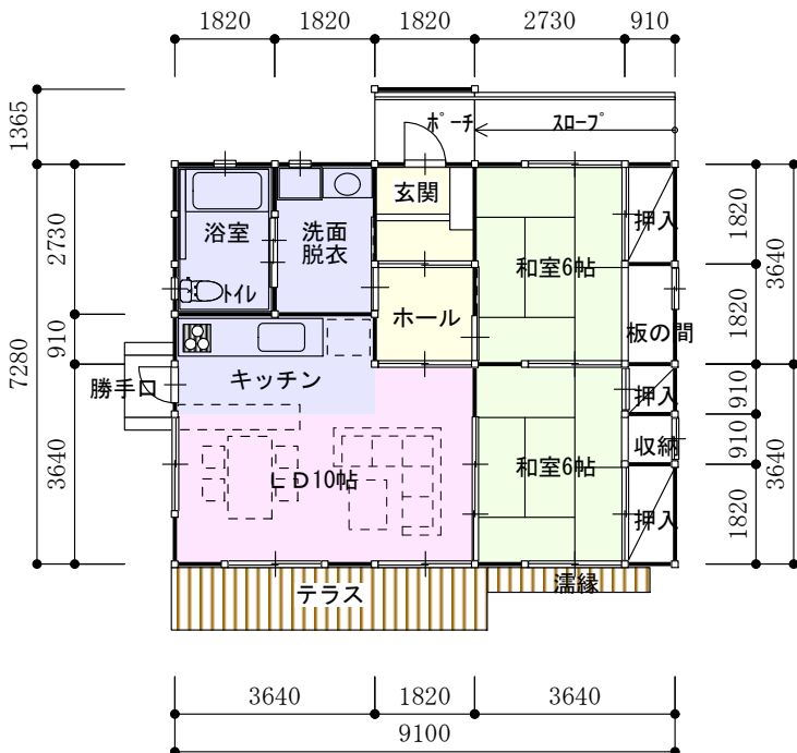
1階平面図 (北入口) S=1/150
