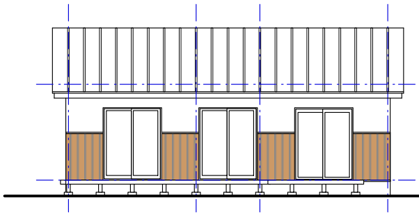
南立面図 S=1/150
