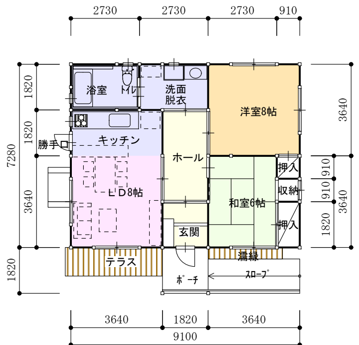
1階平面図 (南入口) S=1/150
